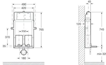
Set de Montaje para Inodoro con Depósito Incorporado
